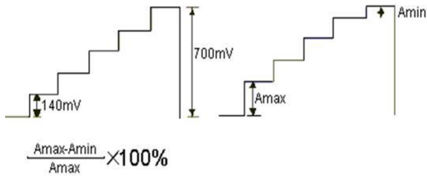
图 14 亮度非线性
