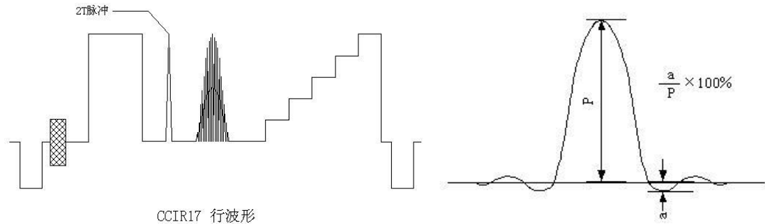
图 13 亮度线性 (K 系数)
