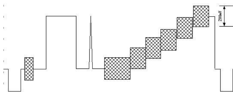
CCIR330 行波形
