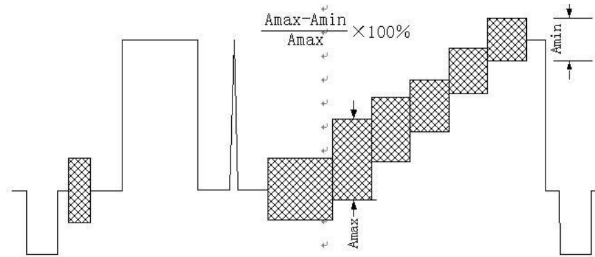
图 15 微分增益
