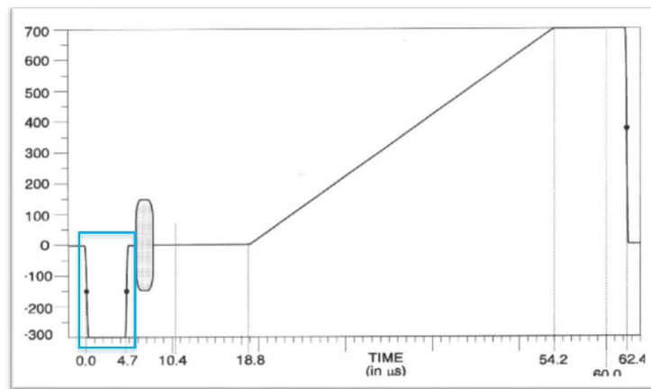
图 6 同步信号
