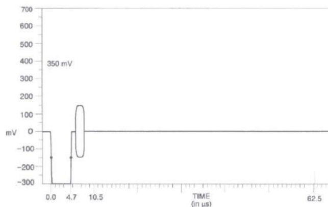
图 20 信噪比
